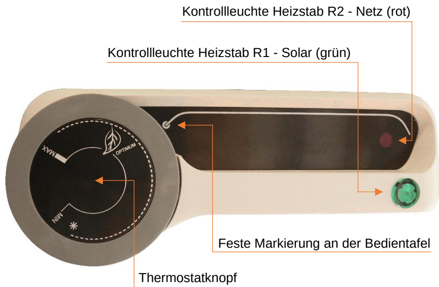
Abbildung 7: Bedienfeld des Warmwasserspeichers
