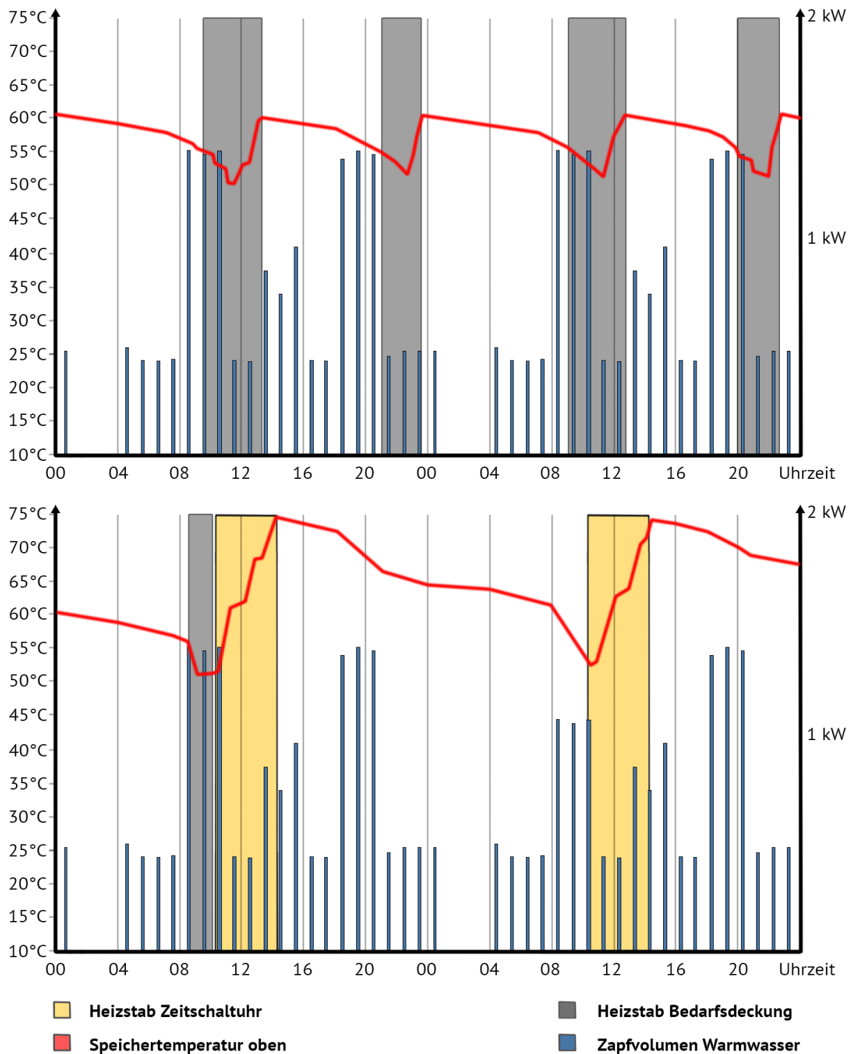
Abbildung 11: Betriebsweise „Bedarfsdeckung“ (oben) und „Solarstromnutzung“ (unten)
